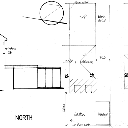
SITE PLAN 1:200
